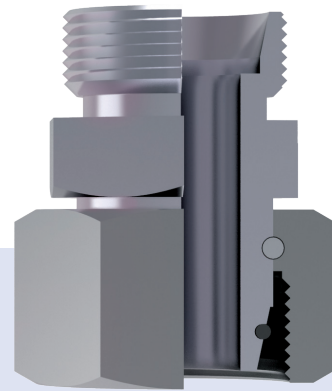
Distanzadapter mit Dichtkegel und O-Ring
